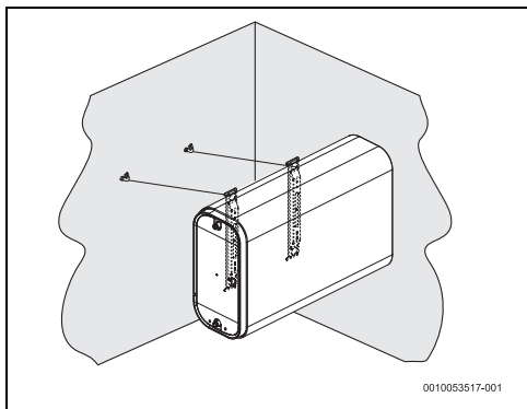
sl. 10 Horizontalna instalacija (zidna montaža)
