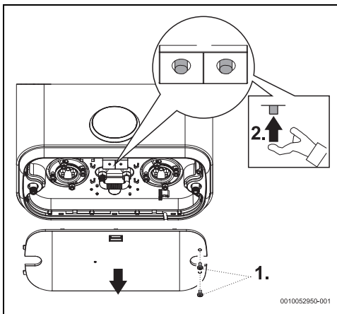
Rys. 15 Termostat zabezpieczający
