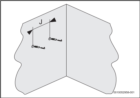
7. ábra Rögzítőcsavarok
