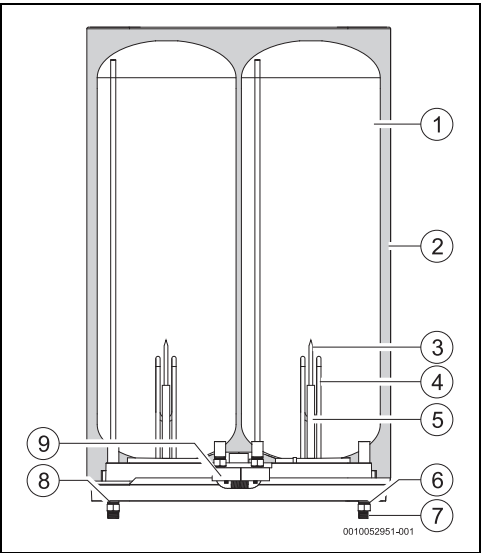
Фиг. 4 Компоненти на уреда
