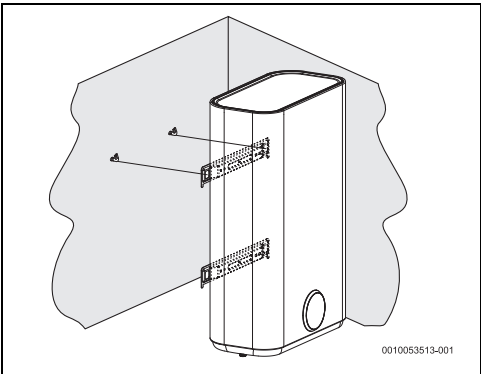
Sl.8 Navpična montaža (pritrditev na steno)
