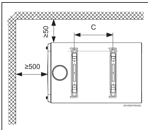
Сл. 3 Димензии во mm (монтажа на сид, хоризонтална инсталација)
