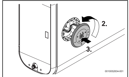
12. ábra A kijelző elfordítása és rögzítése
