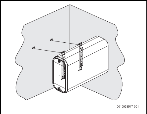
Sl.10 Vodoravna montaža (pritrditev na steno)
