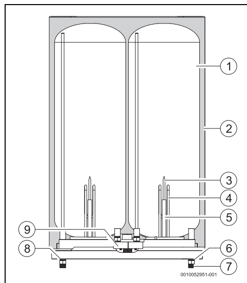
Rys. 4 Komponenty urządzenia
