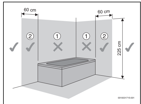
6. ábra Védőzóna
