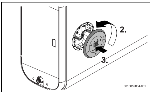
Rys. 12 Obracanie i mocowanie wyświetlacza
