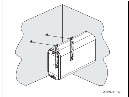
fig. 10 Instalim horizontal (montim në mur)
