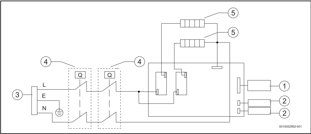
Rys. 16 Schemat połączeń
