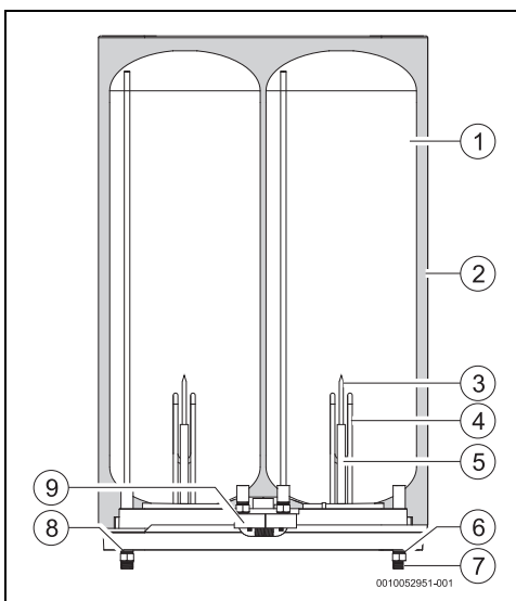
sl. 4 Komponente uređaja
