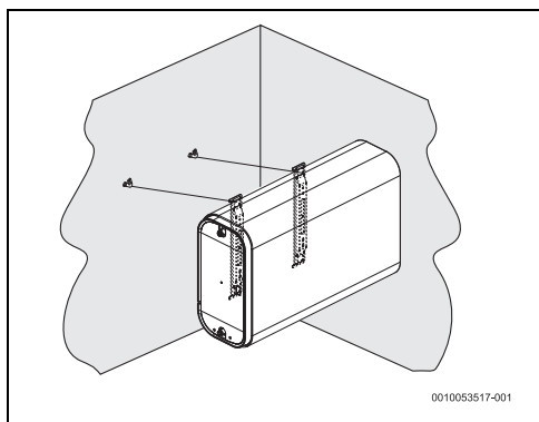
Фиг. 10 Горизонтална инсталация (стенен монтаж)
