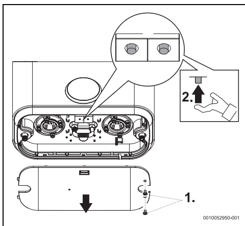
sl. 15 Sigurnosni termostat
