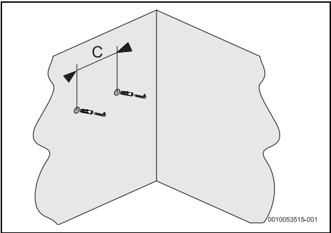
Rys. 9 Śruby mocujące
