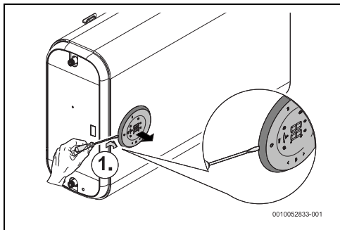
Σχ. 11 Λασκάρισμα οθόνης
