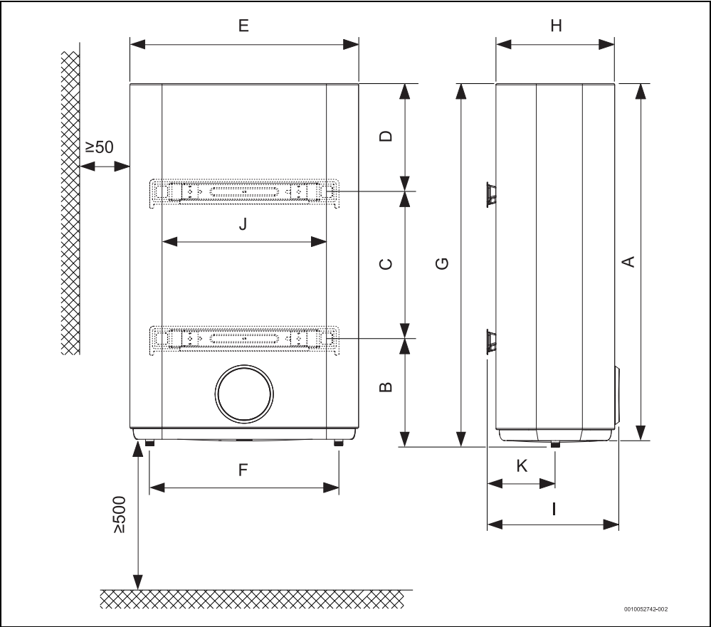
Sl.2 Mere v mm (pritrditve na steno, navpična montaža)
