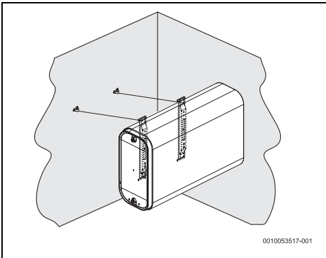
Сл. 10 Хоризонтална инсталација (монтажа на сид)
