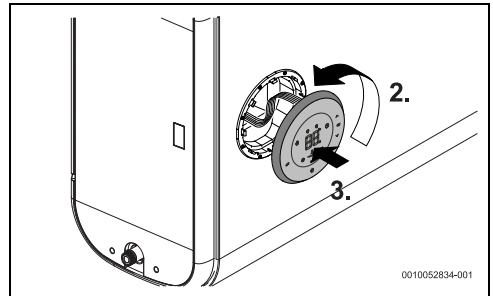
Сл. 12 Завртете го и закачете го приказот
