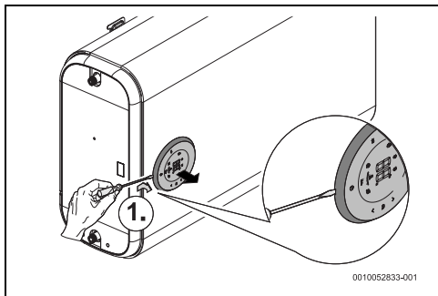
Rys. 11 Odłączanie wyświetlacza
