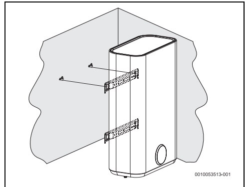
Σχ. 8 Κάθετη εγκατάσταση (επιτοίχια)
