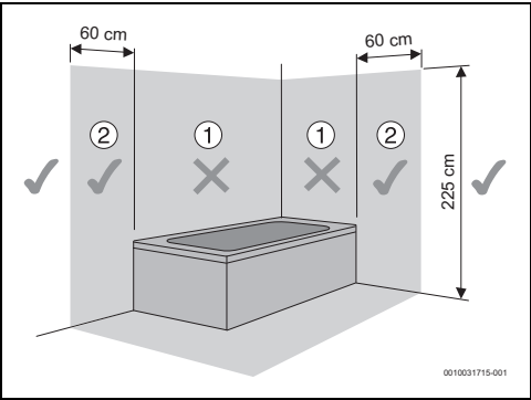
Rys. 6 Strefa ochronna
